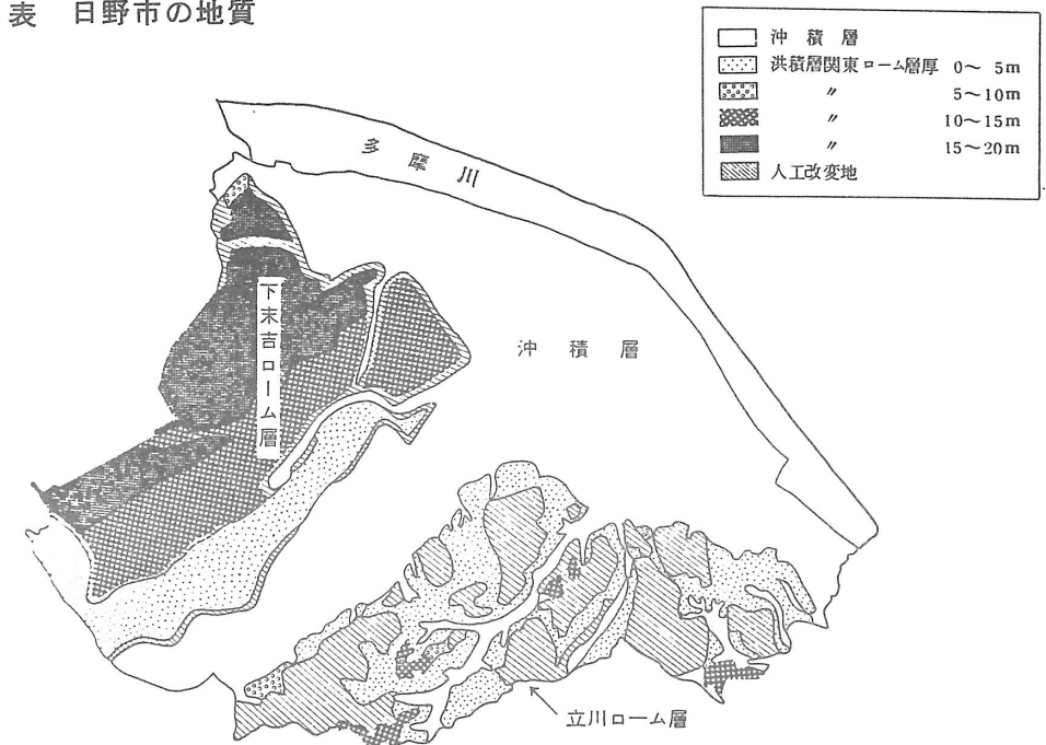
第5表 日野市の地質
