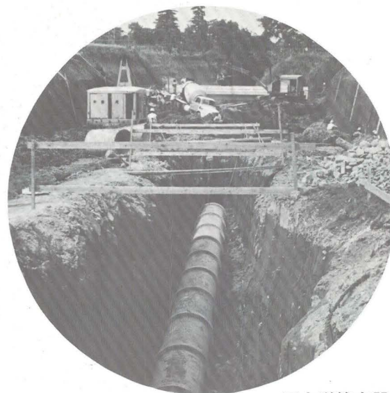
下水道管布設工事
