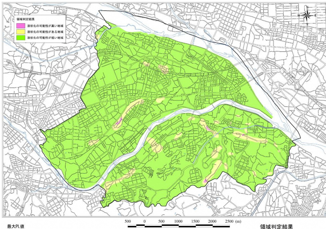
【日野市液状化危険度判定】
