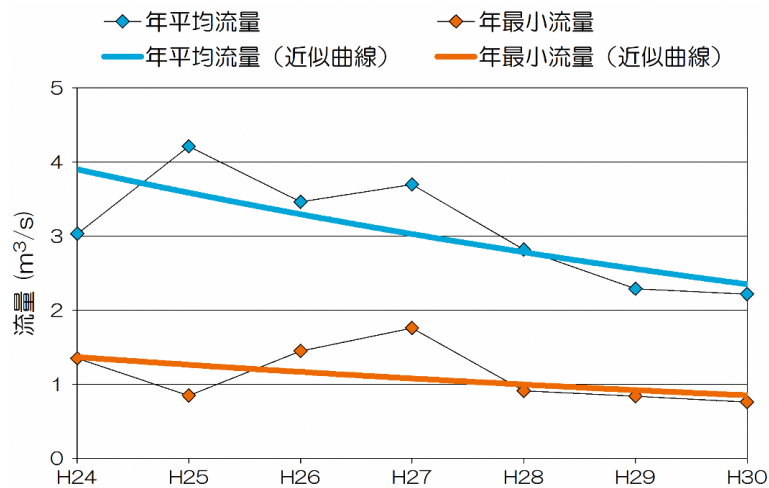
【浅川（高幡橋）における流量の推移】
