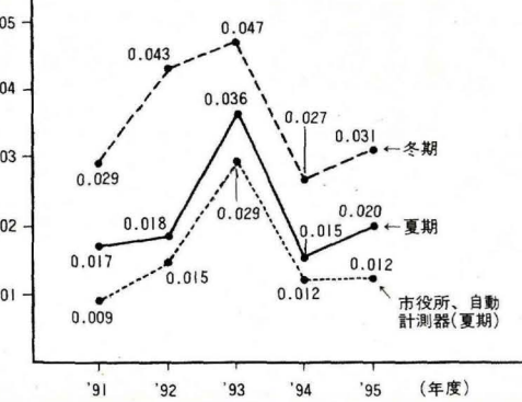
二酸化窒素測定結果平均値の推移
