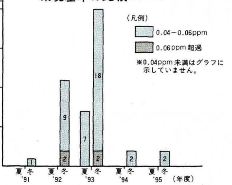
二酸化窒素測定結果平均値の推移
