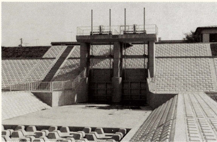
日野樋管（神明上）設置
