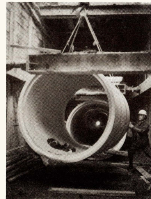
多摩川第 2 排水区管渠埋設
