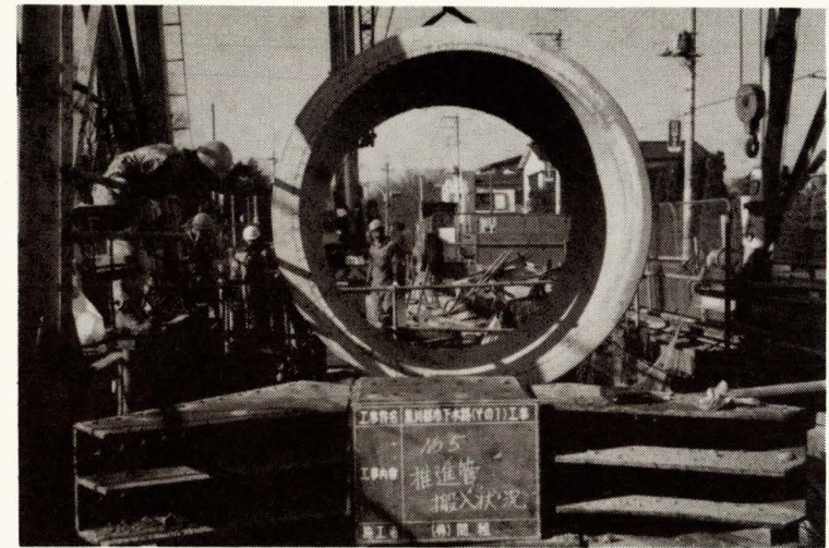
黒川都市下水路管渠埋設
